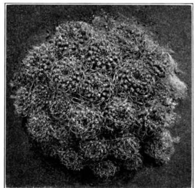
FIG. 223.—Frailea pumila.
